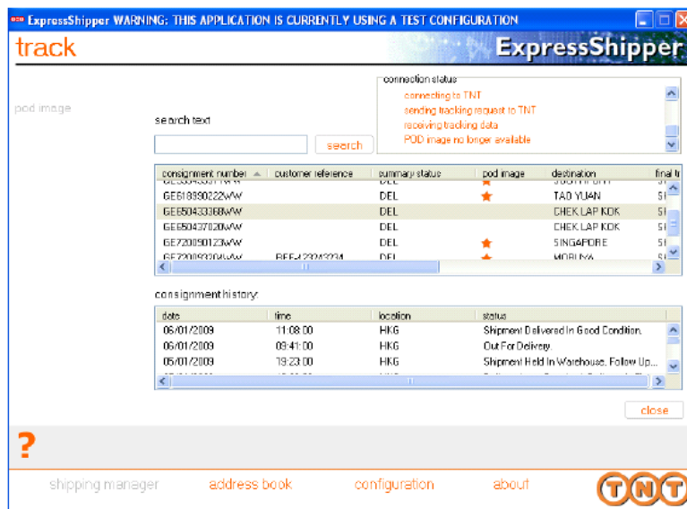
Figuur 13: traceren van zendingen.
