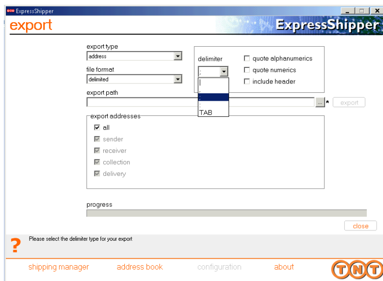
Figuur 18: exporteren van adresgegevens.
